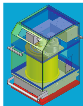
BASICA - řez odprašovačem
